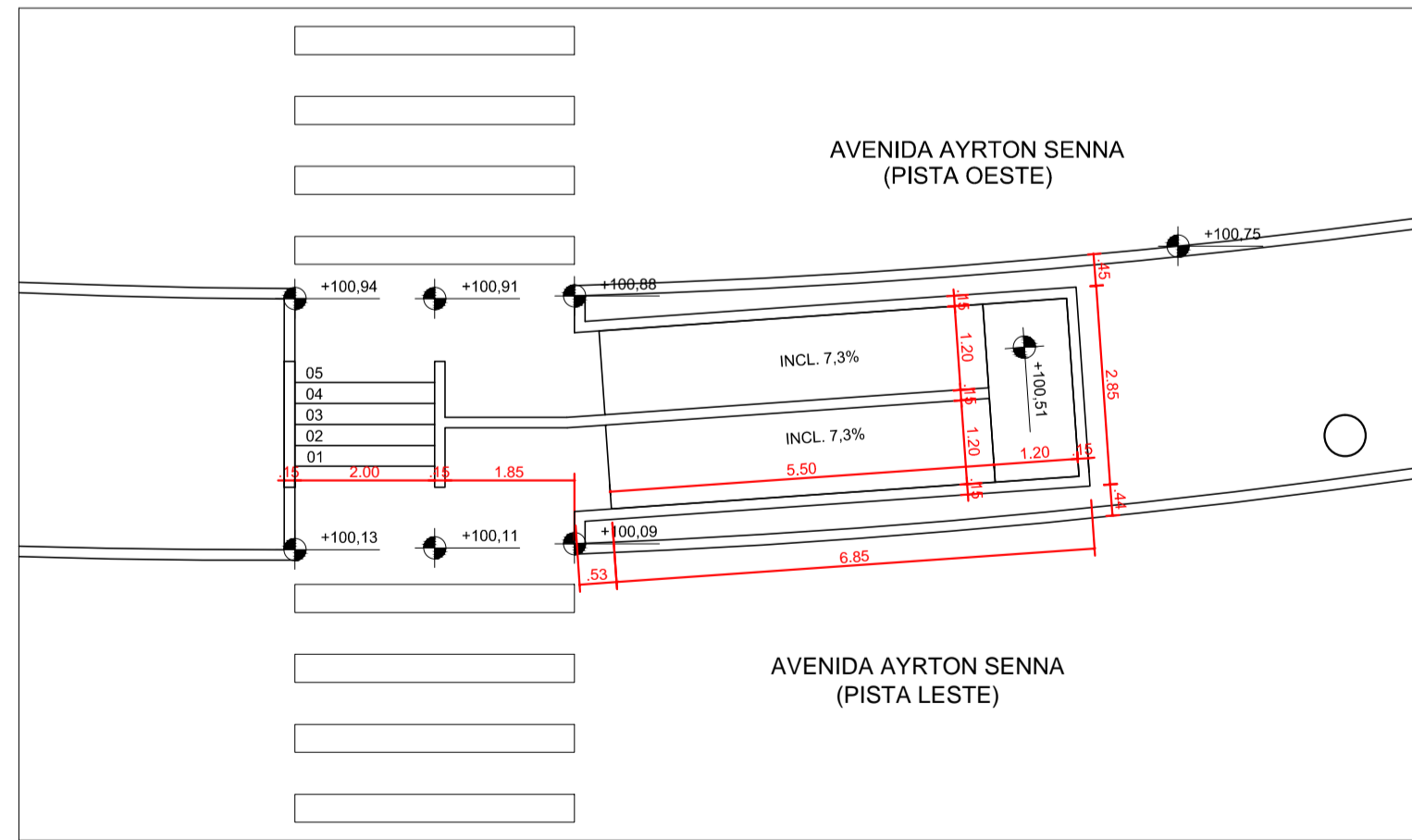
PLANTA – ESCADA E RAMPA PARA CADEIRANTES – VER PLANTA DE DETALHAMENTO escala: 1:100
