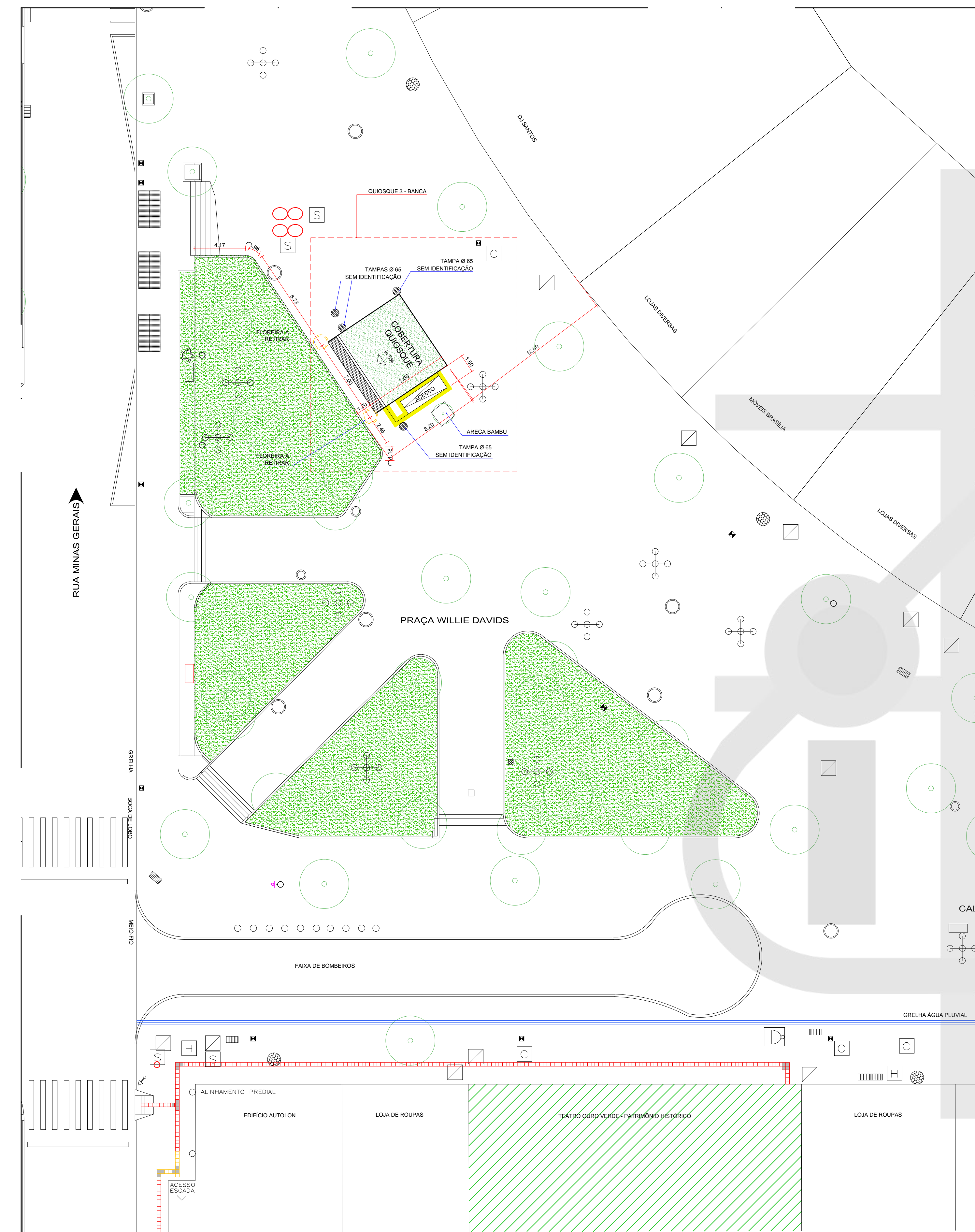
1 IMPLANTAÇÃO - CALÇADÃO EXISTENTE - QUIOSQUE 3 ESCALA 1:200
