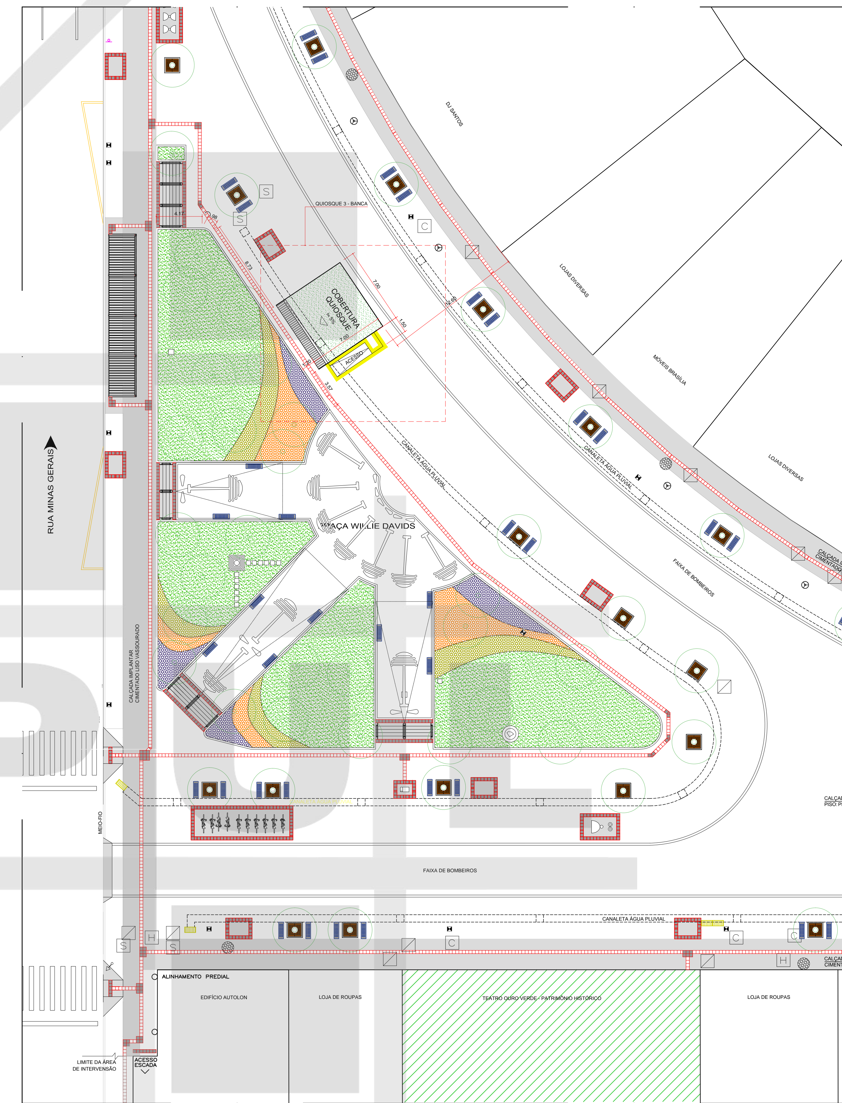
2 IMPLANTAÇÃO - PROJETO REVITALIZAÇÃO CALÇADÃO - QUIOSQUE 3 ESCALA 1:200
